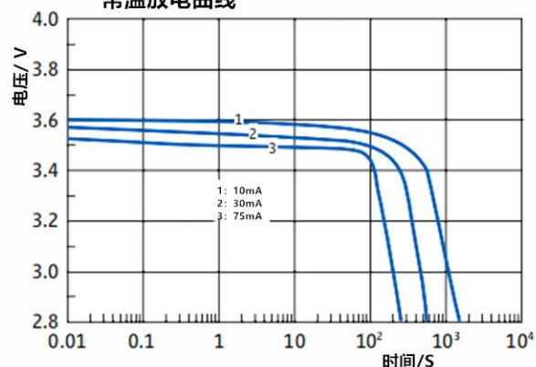
放电电流-时间关系曲线(3.6-2.8V)
