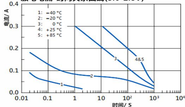
放电电流-时间关系曲线(3.6-2.8V)
