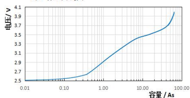
电压-容量曲线图
